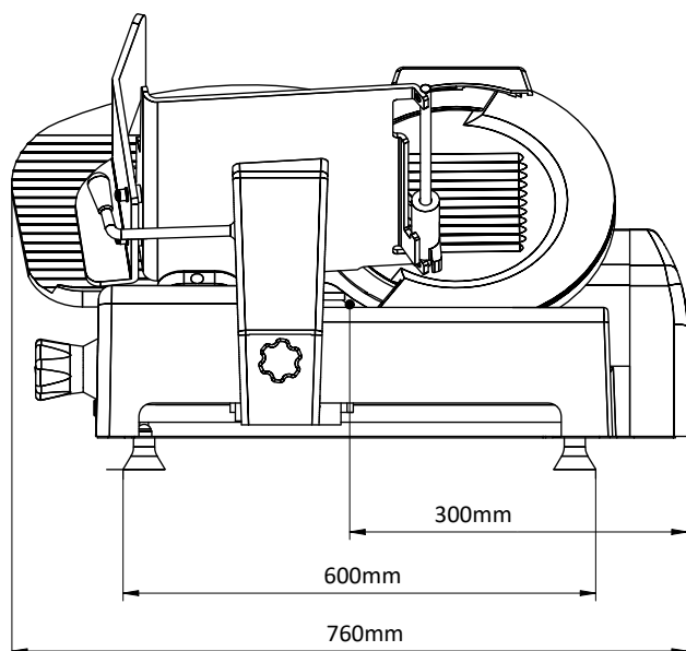
Côté
